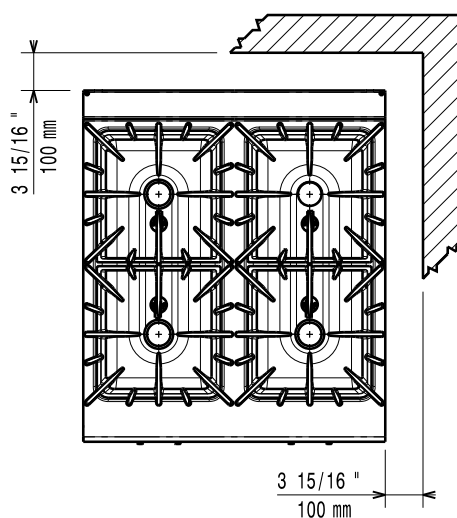
Boven aanzicht
